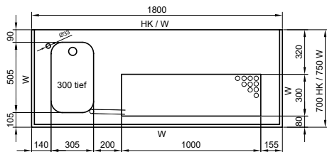
Abdeckung 1800 mm
