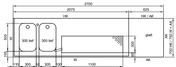
Abdeckung 2700 mm
