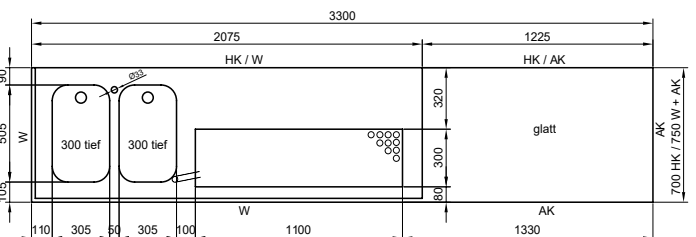
Abdeckung 3300 mm
