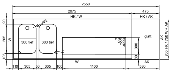
Abdeckung 2550 mm
