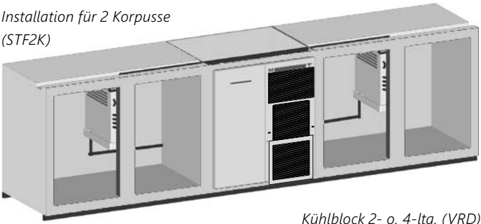
Kühlblock 2- o. 4-ltg. (VRD) statt oder zusätzlich zum Verdampfer
