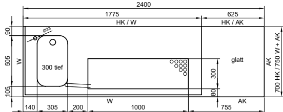
Abdeckung 2400 mm
