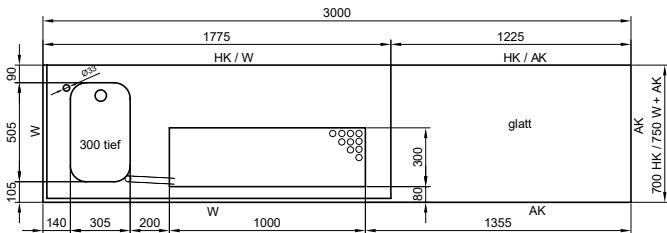
Abdeckung 3000 mm
