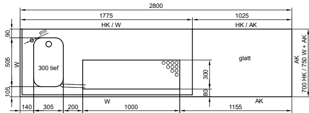
Abdeckung 2800 mm
