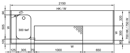
Abdeckung 2150 mm
