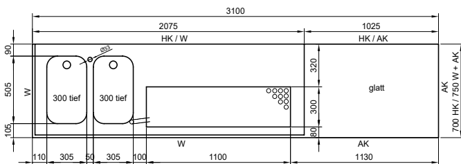
Abdeckung 3100 mm
