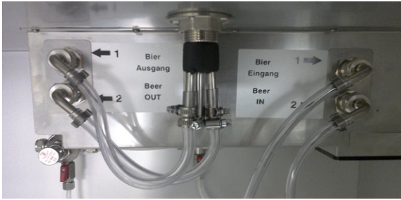
Kühlblock 2- o. 4-ltg. (VRD) statt oder zusätzlich zum Verdampfer
